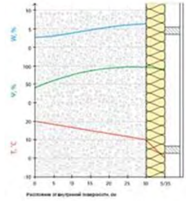
G1 – минвата и облицовка на откосе
