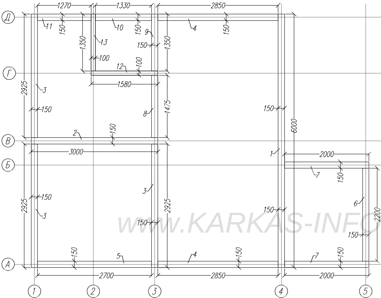
Обвязка стен первого этажа
