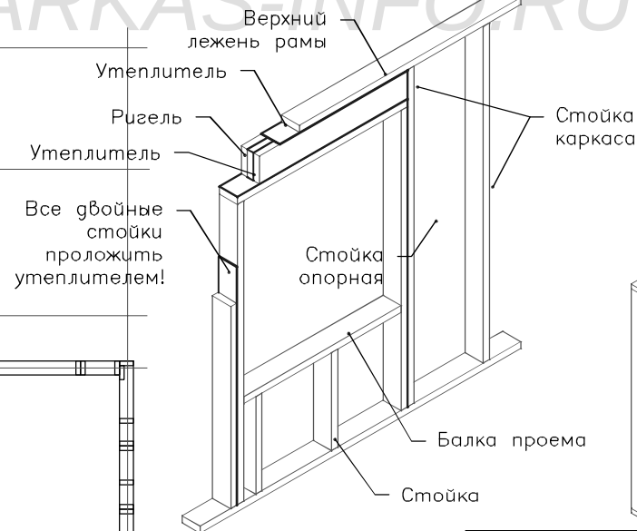
Узел проема оконна/двери.
